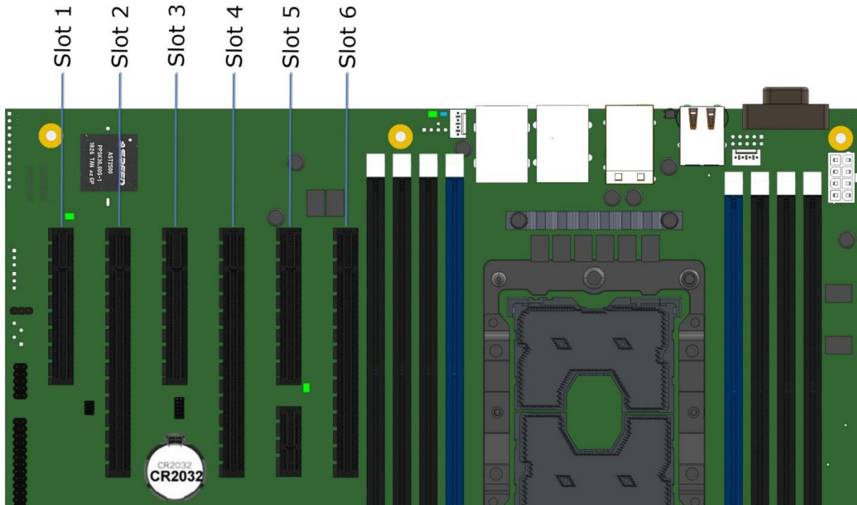
Рисунок 69. Слоты PCIe*
