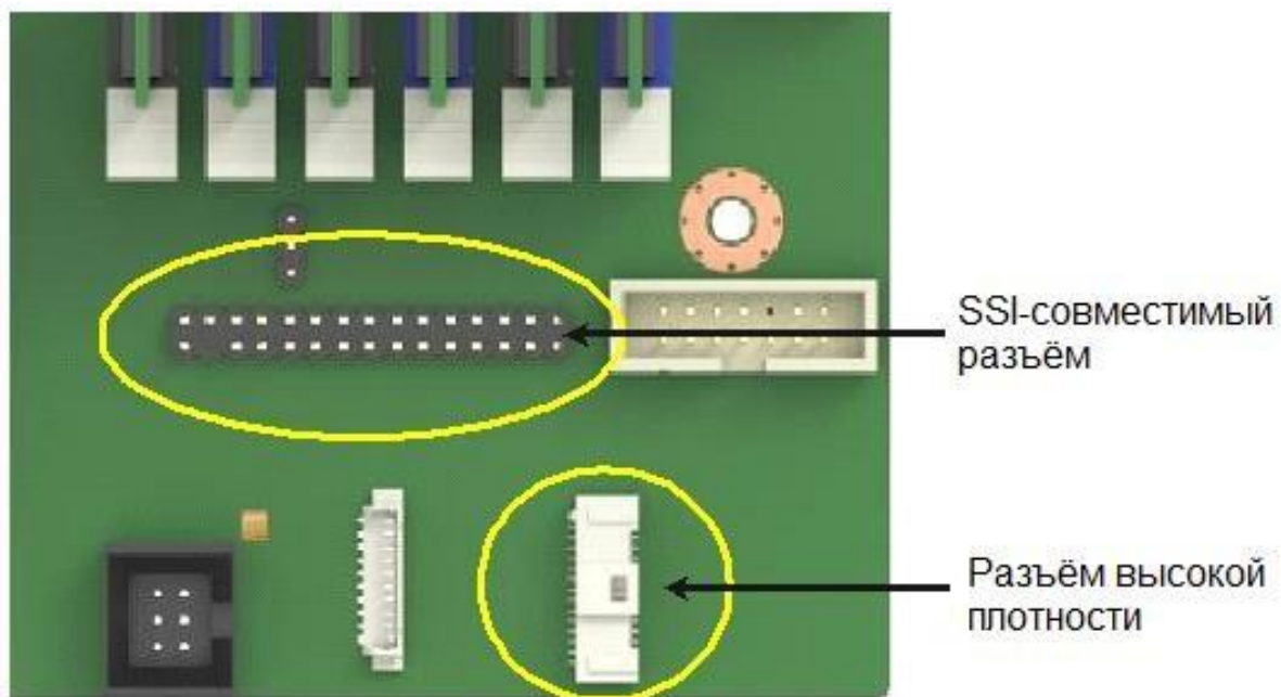
Рисунок 50. Варианты разъёмов
