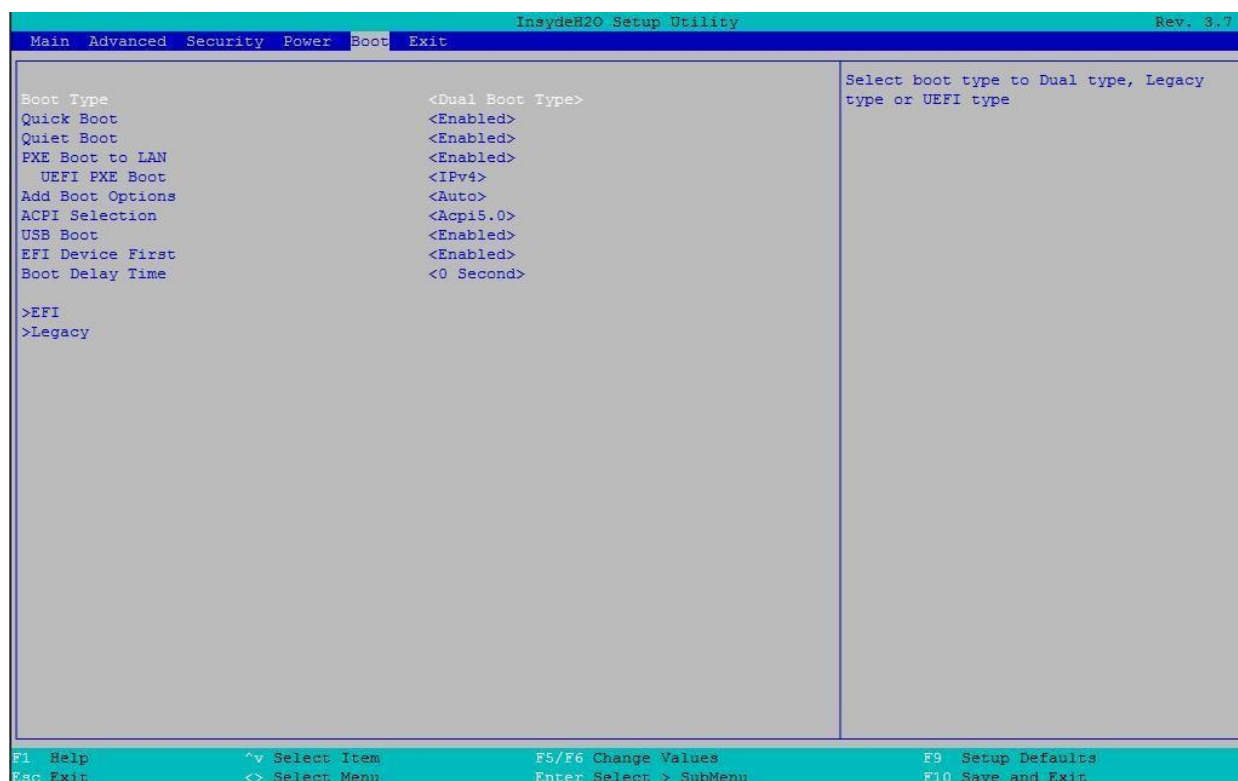
Рисунок 131. Загрузочное меню
