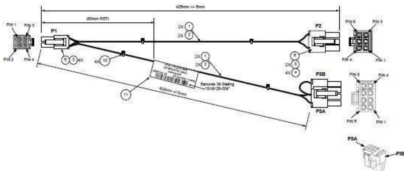
Рисунок 49. Дополнительный кабель питания на 12 В
