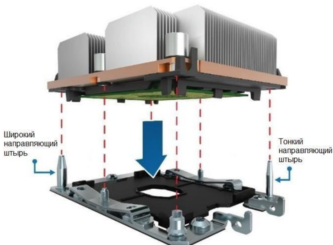
Рисунок 19. Монтаж процессора на разъём платы
