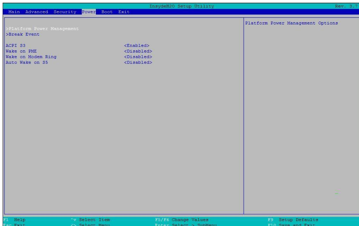
Рисунок 128. Меню электропитания
