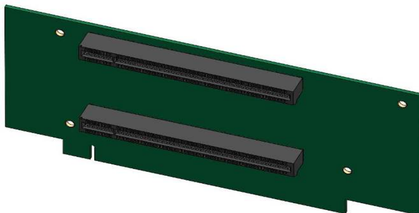
Рисунок 28. 2-х портовая (x16 и x16) 2U переходная плата (469535.082)
