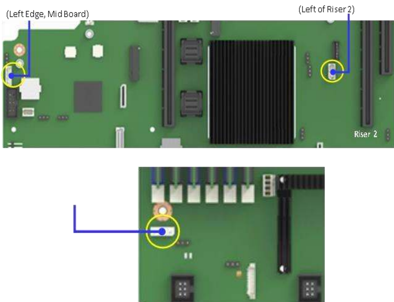
Рисунок 56. Местоположение разъемов I2C объединительной платы
